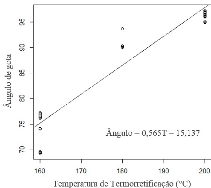
FIGURA 3: Gráfico da regressão linear do ângulo de gota em função da temperatura de termorretificação.
