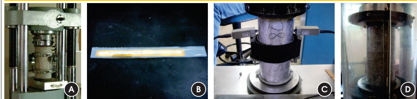
Figure 2 – Dial Indicators (a) Strain gage (b), Clip gage (c) and LVDT (d)
