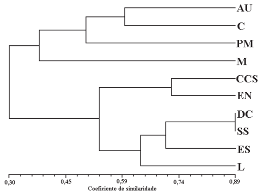
Figura 2 – Dendrograma obtido através do método hierárquico de agrupamento UPGMA com base na similaridade florística (coeficiente de similaridade de Jaccard), para Baccharis sect. Caulopterae (Asteraceae) entre as regiões fisiográficas do Rio Grande do Sul: Alto Uruguai (AU), Campanha (C), Campos de Cima da Serra (CCS), Depressão Central (DC), Encosta do Nordeste (EN), Encosta do Sudeste (ES), Litoral (L), Missões (M), Planalto Médio (PM) e Serra do Sudeste (SS).
