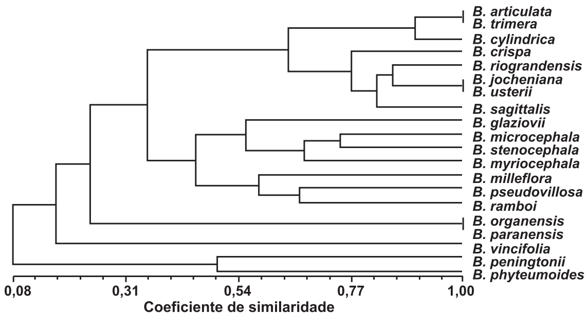
Figura 4 – Dendrograma obtido através do método hierárquico de agrupamento UPGMA ( Unweighted Pair Group Main Average ) com base na similaridade de distribuição geográfica (coeficiente de similaridade de Jaccard) das espécies de Baccharis sect. Caulopterae (Asteraceae) ocorrentes no Rio Grande do Sul.
