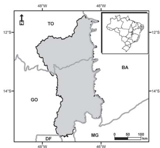
Figura 1 – Localização geográfica da bacia do rio Paranã (em cinza) nos estados de Goiás e Tocantins.
