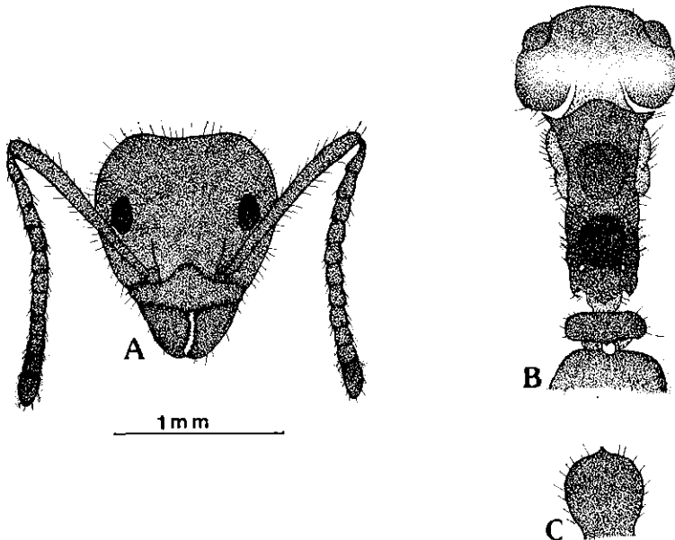
Fig. 2. Monacis inpai n. sp. Holótipo, operária. A - cabeça em vista frontal; B - alitrongo em vista dorsal; C - vista anterior da escama do pecíolo.
