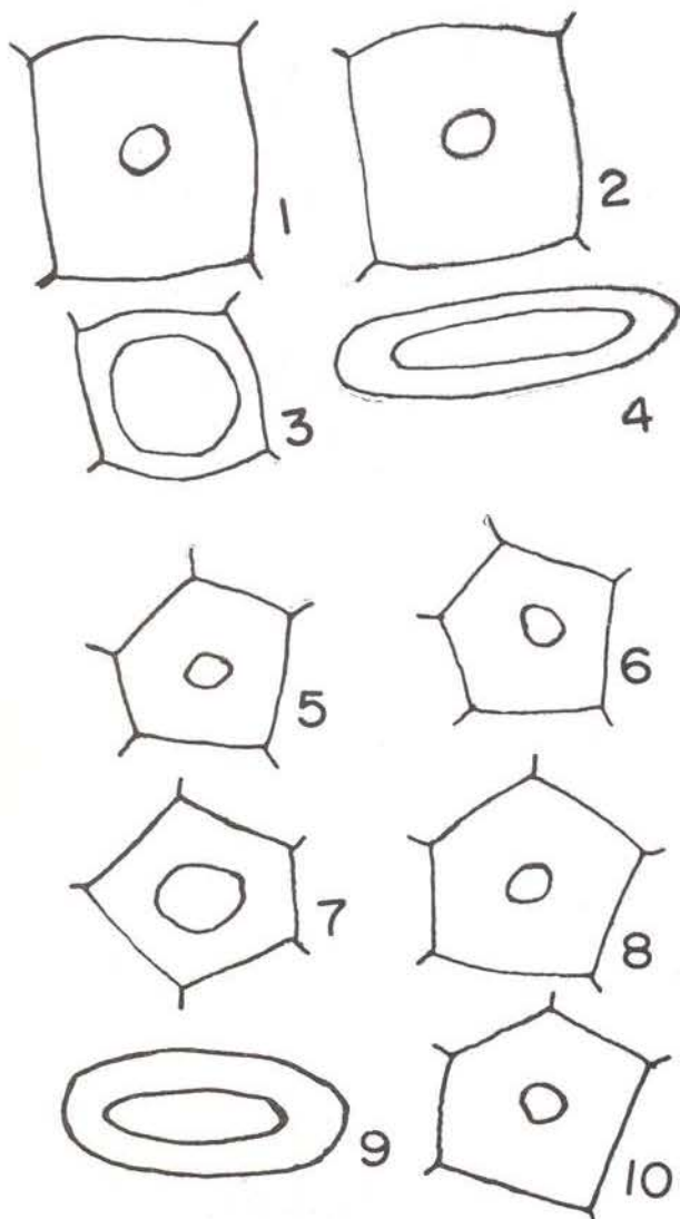
Fig. 1 — Catostemma commune : aspecto da fibra dentro da madeira. Fig. 2 — Catostemma commune : aspecto da fibra dentro do papel. Fig. 3 — Scleronema micranthum : aspecto da fibra dentro da madeira. Fig. 4 — Scleronema micranthum : aspecto da fibra dentro do papel. Fig. 5 — Catostemma sclerophyllum : aspecto da fibra dentro da madeira. Fig. 6 — Catostemma sclerophyllum : aspecto da fibra dentro do papel. Fig. 7 — Catostemma milanezii : aspecto da fibra dentro da madeira. Fig. 8 — Catostemma milanezii : aspecto da fibra dentro do papel. Fig. 9 — Catostemma albuquerquei : aspecto da fibra dentro da madeira. Fig. 10 — Catostemma albuquerquei : aspecto da fibra dentro do papel.
