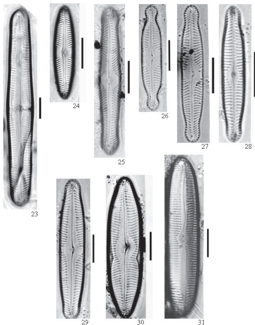
Figura 23. Pinnularia macilent a (Ehrenberg) Ehrenberg. 24. P. schoenfelderi Krammer. 25. P. similis Hustedt. 26. P. subanglica Krammer. 27. P. subcapitata Gregory var. elongata Krammer. 28. P. subcapitata Krammer var. semicruciat a Metzeltin & Lange-Bertalot. 29. P. subgibba Krammer. 30. P. variarea Metzeltin & Krammer. 31. P. viridiformis Krammer var. minor Krammer. Barras: 10 \mu\text{m} .
