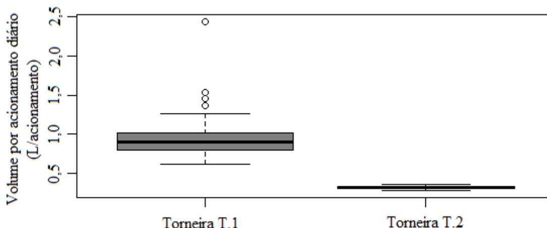
Figura 7 - Boxplots dos dados de volume por acionamento diário para as torneiras convencional (T.1) e de funcionamento hidromecânico (T.2)
