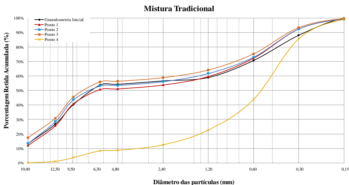
Figura 7 - Curva granulométrica da mistura tradicional - betoneira de eixo inclinado
