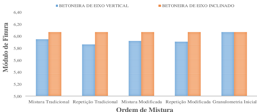
Figura 9 - Valores de módulo de finura dos agregados graúdos antes e após a mistura
