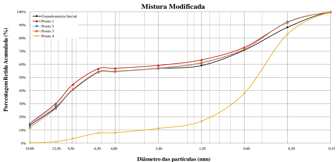
Figura 8 - Curva granulométrica da mistura modificada - betoneira de eixo inclinado
