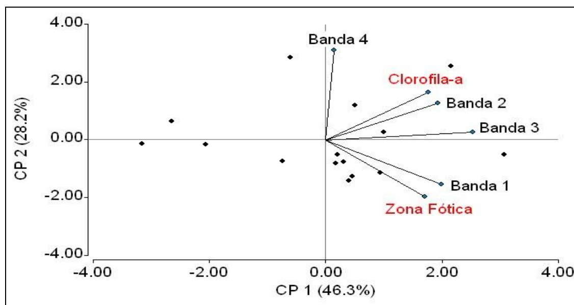
Figura 2. Diagrama de Componentes Principales (CPI/CP2).
