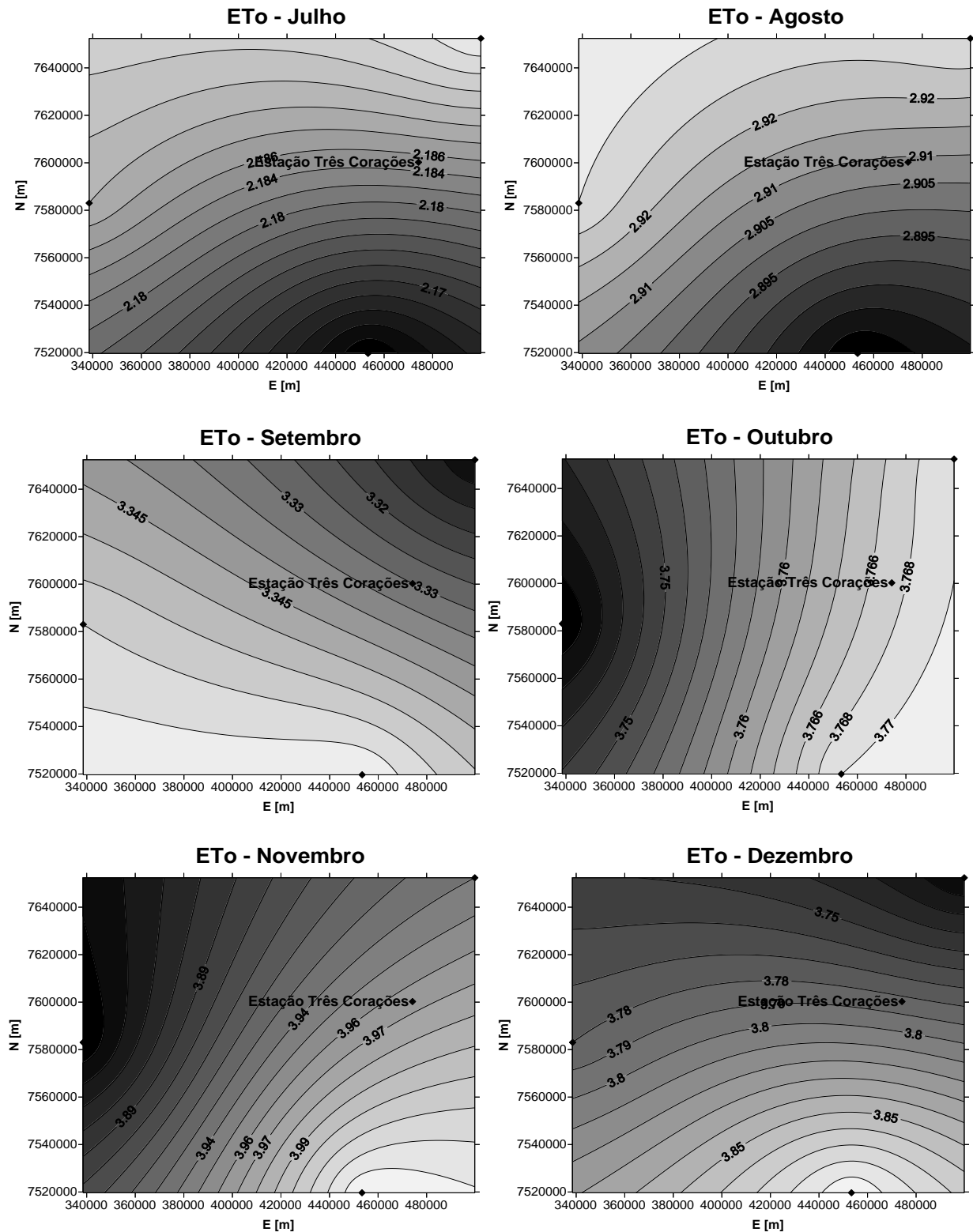
Figura 5. Evapotranspiração de referência média mensal interpolada por krigagem para os meses de julho a dezembro (1975 a 2000).
