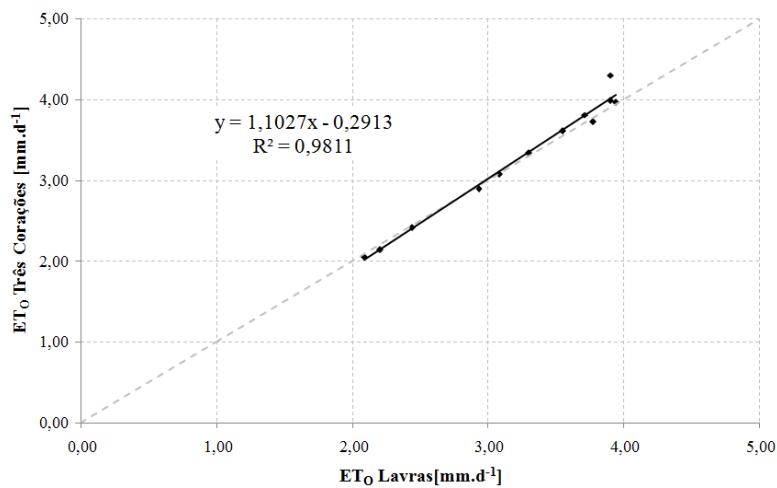
Figura 2. Regressão linear entre as evapotranspirações de referência médias mensais da estação Três Corações e a estação Lavras.
