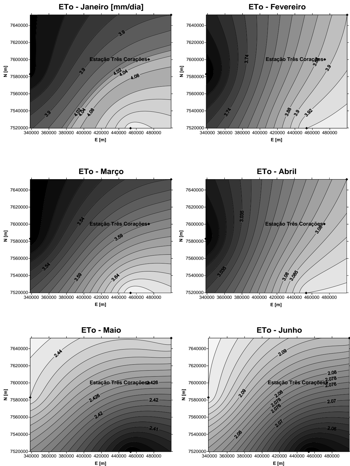
Figura 4. Evapotranspiração de referência média mensal interpolada por krigagem para os meses de janeiro a junho (1975 a 2000).
