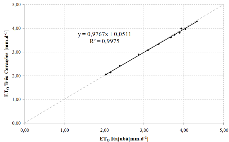
Figura 1. Regressão linear entre as evapotranspirações de referência médias mensais da estação Três Corações e a estação Itajubá.
