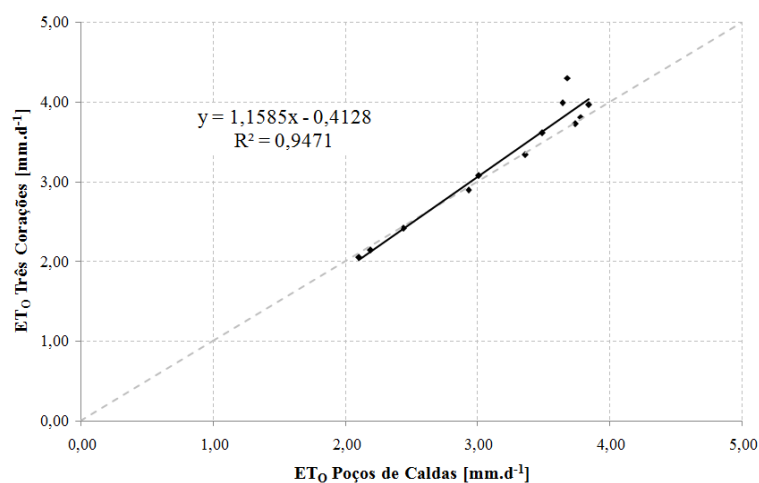
Figura 3. Regressão linear entre as evapotranspirações de referência médias mensais da estação Três Corações e a estação Poços de Caldas.
