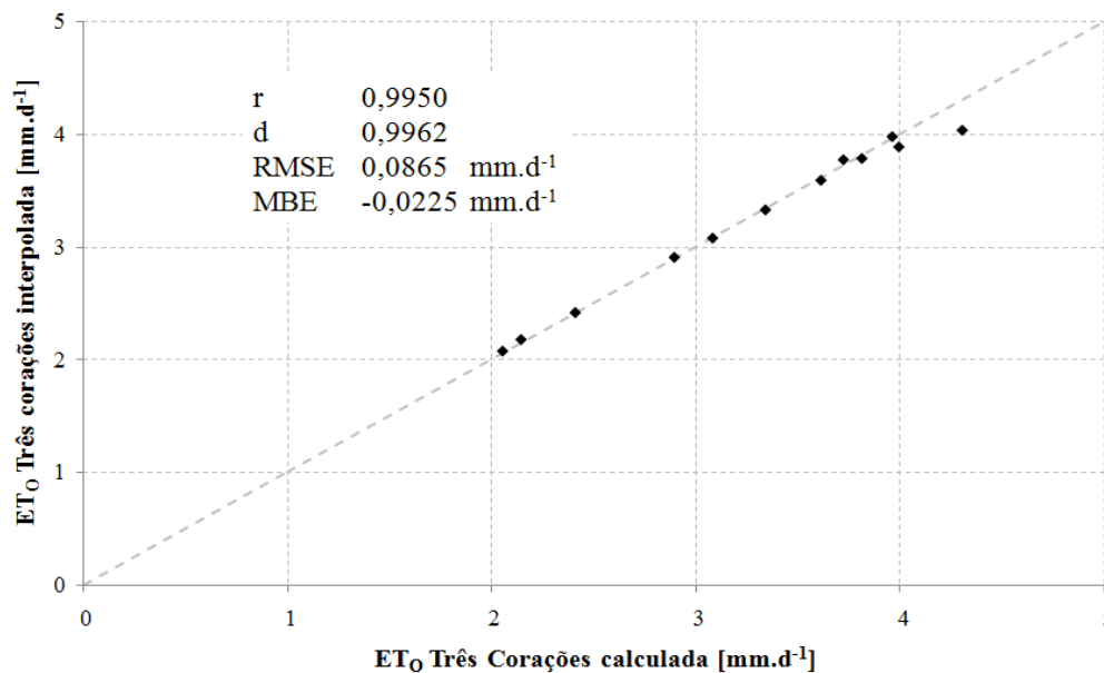
Figura 6. Evapotranspirações de referência médias mensais calculadas e interpoladas para a estação Três Corações.
