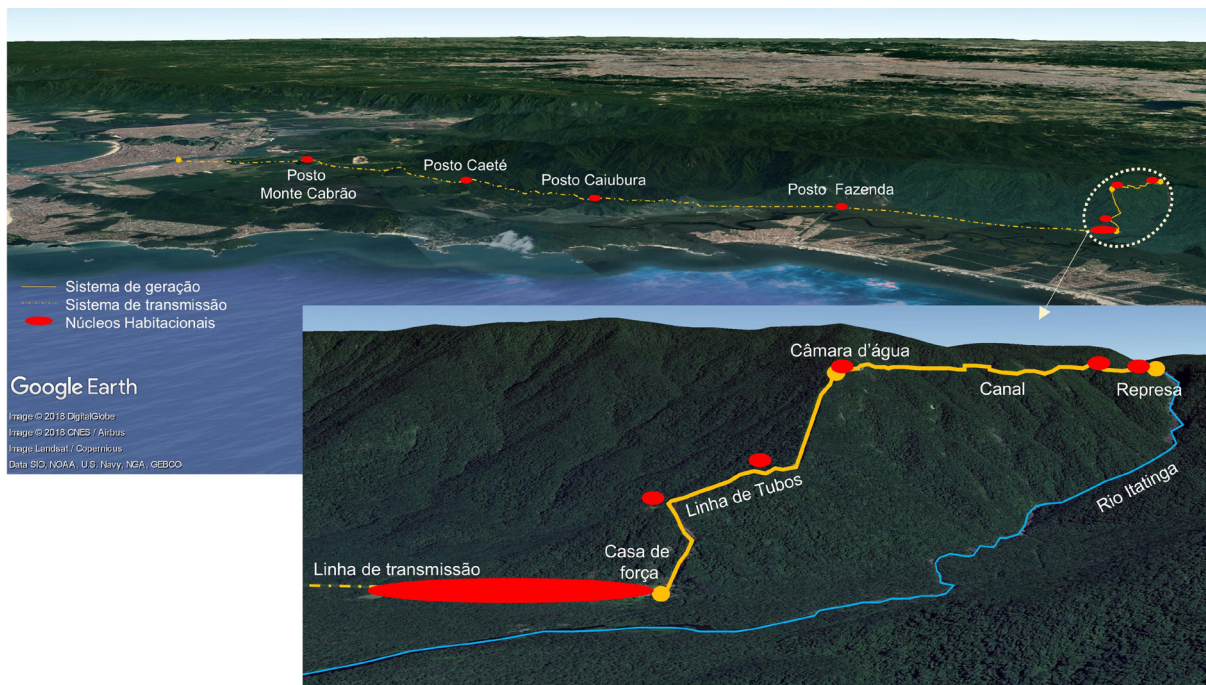
Figura 4 – Usina de Itaipu, 2016. Fonte: Google Earth (adaptado pela autora).
