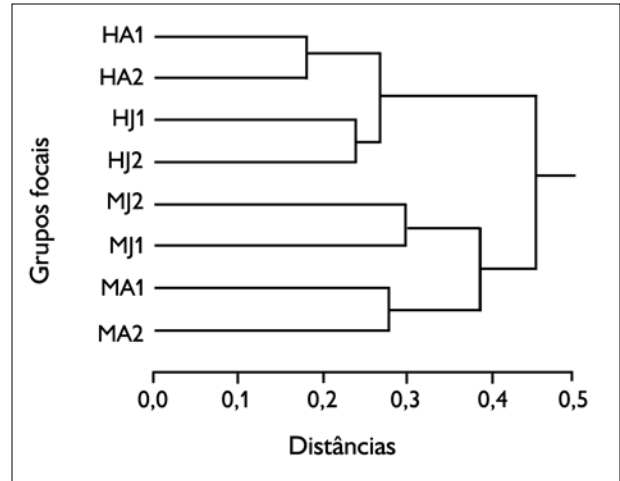
Figura 14. Dendrograma de similaridade (Índice de Jaccard) entre as listas de animais citados por grupos de moradores de Tapiíra, separados por gênero e geração.
