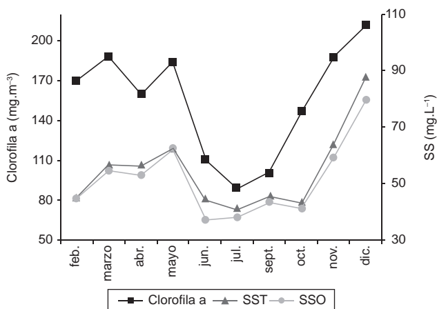
Figura 4. Variación de la concentración de clorofila a (mg.m -3 ) y del contenido de sólidos suspendidos totales y de origen orgánico (mg.L -1 ), en la laguna Don Tomás, entre febrero y diciembre de 2006.
