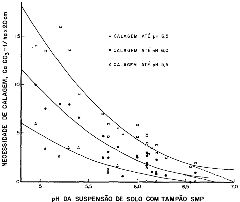
Figura 2. - Necessidade de calagem de solos com base na depressão do pH da solução SMP, para valores de pH dos solos de 5,5, 6,0 e 6,5. As curvas valem para a relação solo:água:solução SMP de 10:20:10; e equações correspondentes apresentadas no quadro 3
