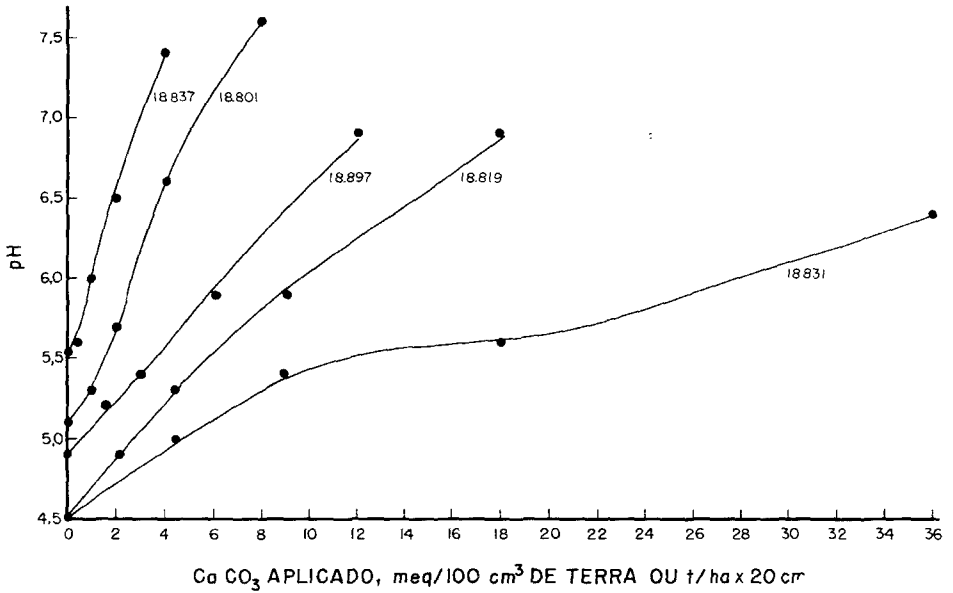
Figura 1. - Curvas de neutralização de cinco amostras de solos com \text{CaCO}_3 . 18.837 - regossolo; 18.801 - latossolo vermelho-amarelo, fase arenosa; 18.897 - latossolo vermelho-amarelo, húmico; 18.819 - latossolo vermelho-escuro, orto; 18.831 - solo com B câmbico
