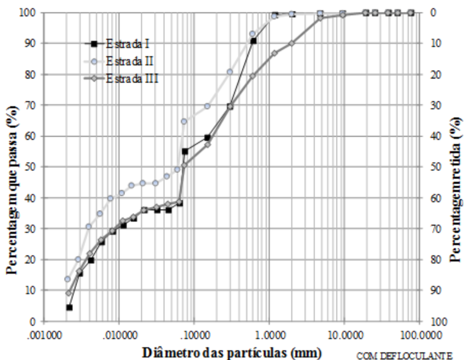
FIGURA 1. Curvas granulométricas de cada trecho das estradas avaliadas. Grain size distribution curves of each evaluated road section.
