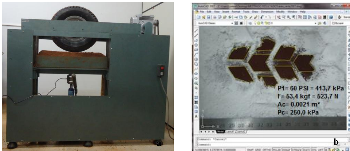
FIGURA 3. a) Vista frontal do simulador linear de tráfego. b) Área de contato do pneu do simulador. a) Traffic simulator front view. b) Tire simulator contact area.
