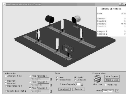
Figura 3. Interferência em regime quântico
