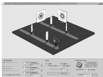
Figura 2. Interferência em regime clássico: padrão de anéis
