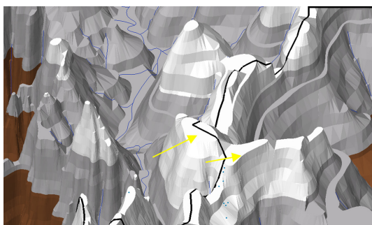
Figura 12. Relevo patamarizado, influência direta na ocorrência de hidromorfia.
