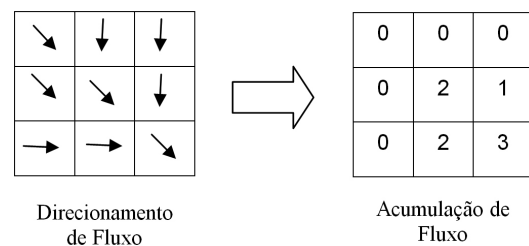
Figura 4. Acumulação de fluxo. Adaptado de Tarboton et al. (1991) e Jenson & Domingue (1988).
