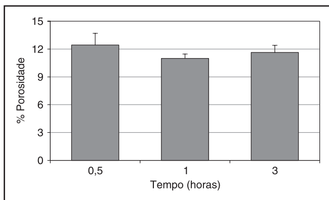
GRÁFICO 2 - Porcentagem de porosidade de amostras de hidroxiapatita sinterizadas por diferentes intervalos de tempo a 1.250^\circ\text{C} . Dados mostrados como média \pm desvio-padrão ( n = 5 ).
