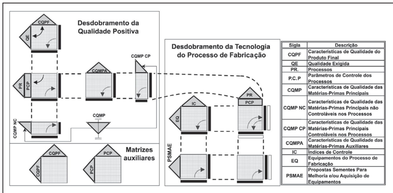
Figura 4: Modelo conceitual.
