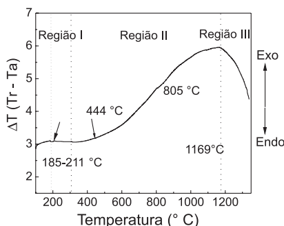
Figura 2. Curva de análise térmica diferencial da fase \text{KSn}_2\text{Nb}_5\text{O}_{15}
