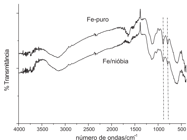
Figura 1. Espectroscopia de infravermelho dos materiais: Fe/Nb (óxido de ferro/óxido de níobia) e Fe-puro (óxido de ferro)
