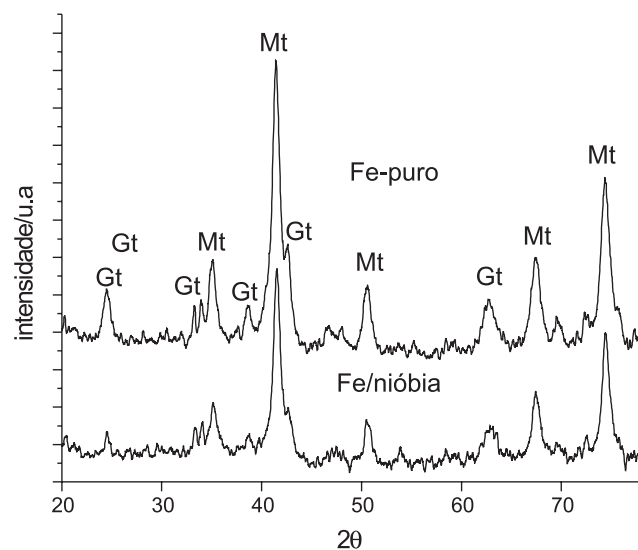
Figura 2. Difratograma de raios-X dos materiais: Fe/Nb (óxido de ferro/óxido de níobia) e Fe-puro (óxido de ferro)
