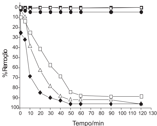
Figura 6. Cinética de remoção da cafeína utilizando os diferentes sistemas de oxidação e dos materiais Fe/Nb (óxido de ferro/óxido de nióbia) e Fe-puro (óxido de ferro) como catalisador ( [I]_{inicial} = 7,76 \text{ mmol L}^{-1} ). ■ = h\nu , ● = \text{H}_2\text{O}_2 + \text{Fe-puro} , ○ = \text{H}_2\text{O}_2 + \text{Fe/Nb} , □ = \text{H}_2\text{O}_2 + \text{Fe-puro} + h\nu , △ = \text{H}_2\text{O}_2 + h\nu , ◆ = \text{H}_2\text{O}_2 + \text{Fe/Nb} + h\nu
