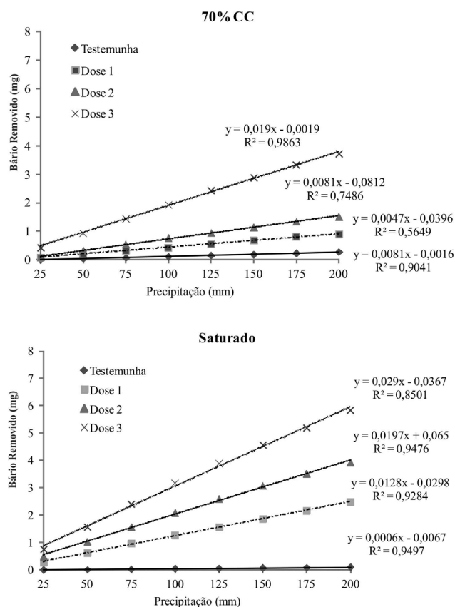
Figura 2. Quantidade de bário (mg) removido em cada volume em função da doses e condições de umidade
