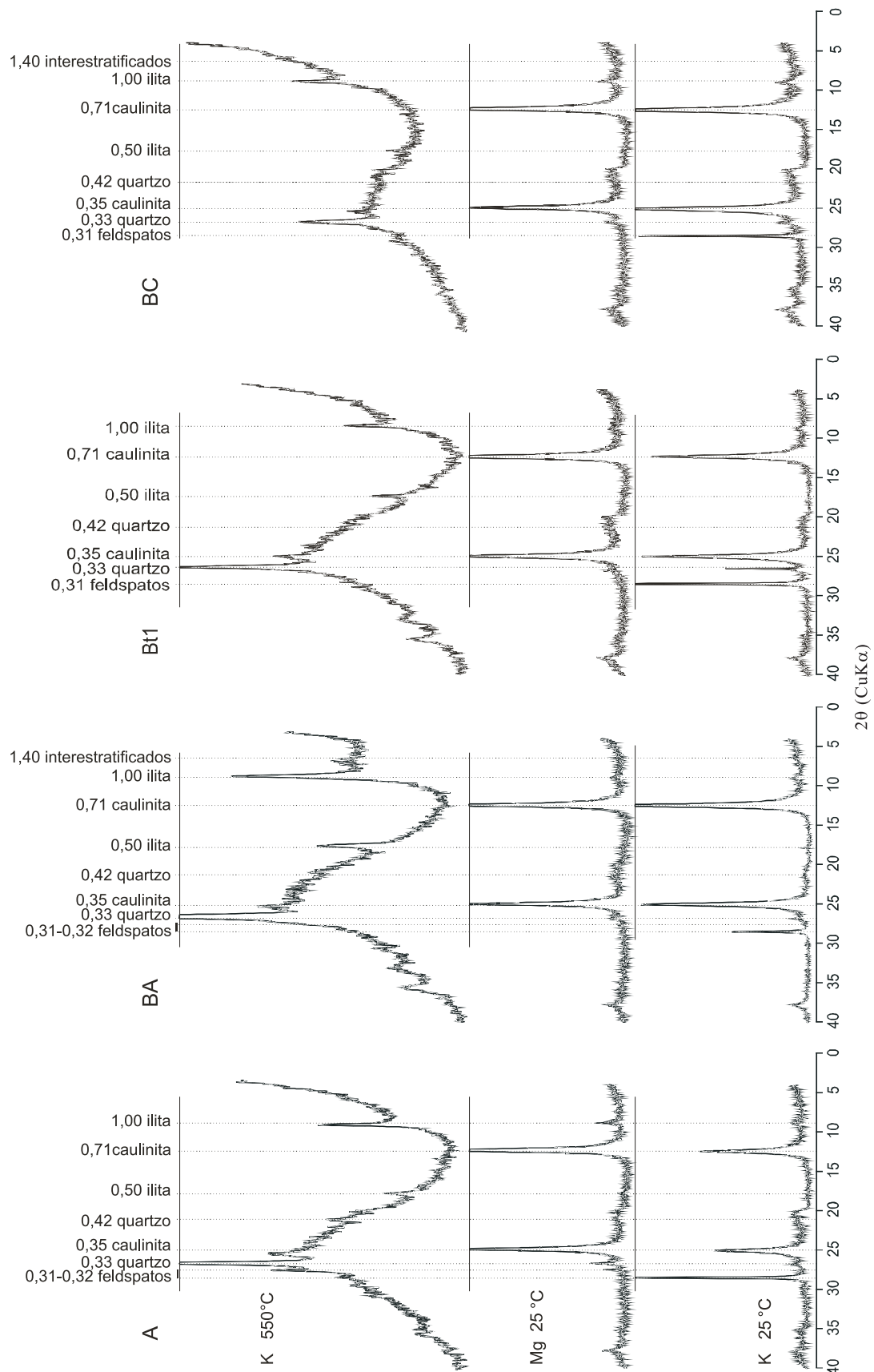
Figura 3. Difratomogramas de raios X dos três tratamentos utilizados da fração argila do Argissolo Vermelho-Amarelo (horizontes A, BA, Bt1 e BC).
