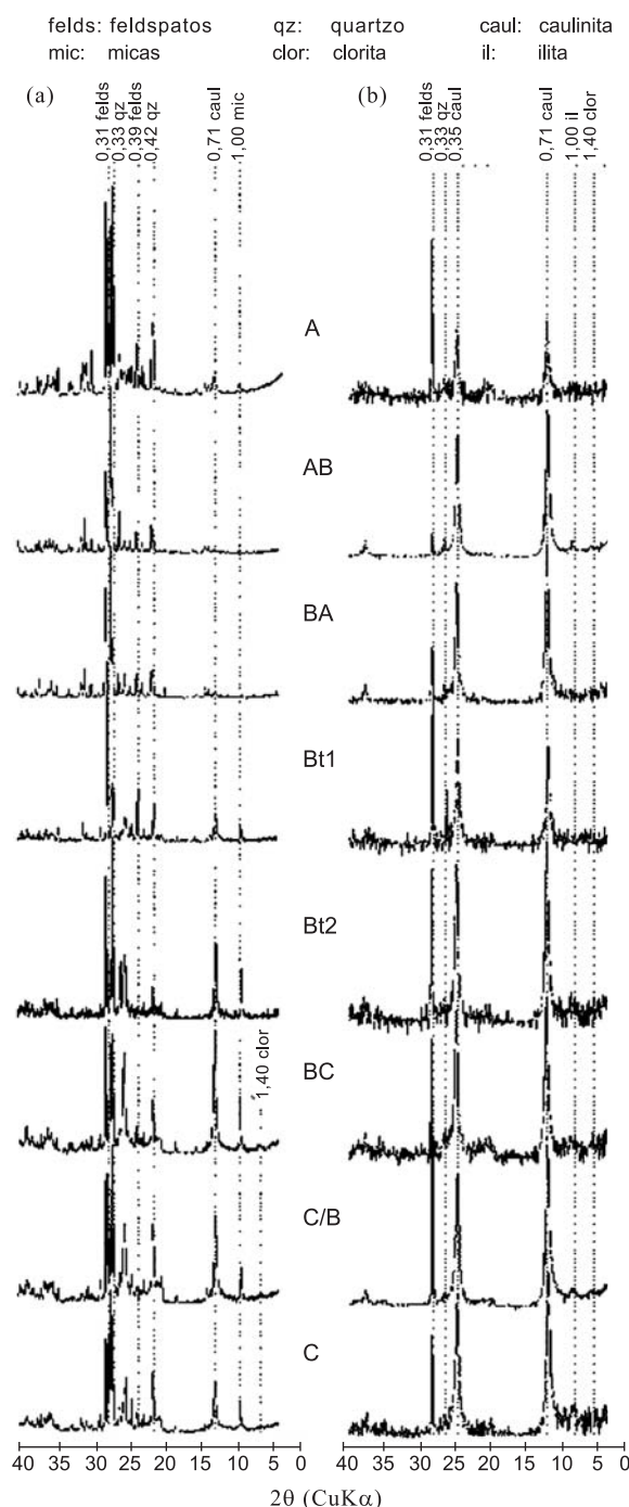
Figura 1. Difratogramas de raios X de K 25°C de todos os horizontes do Argissolo Vermelho-Amarelo: (a) fração silte e (b) fração argila.
