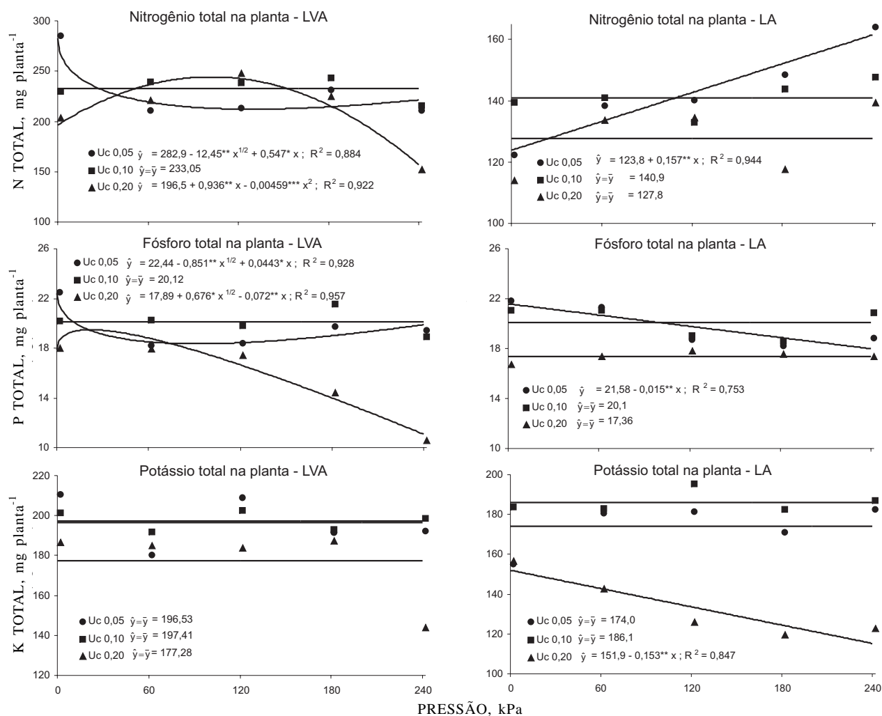
Figura 3. Conteúdos de nitrogênio, fósforo e potássio na matéria seca total de eucalypto em dois Latossolos compactados com diferentes pressões e umidades.
