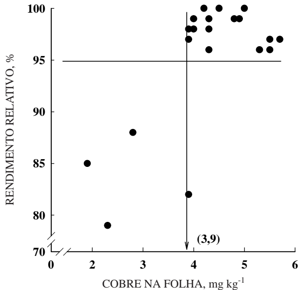
Figura 2. Relação entre rendimentos relativos de grãos a 0,13 kg kg -1 de umidade da soja e teores de cobre extraídos da folha, do segundo e do terceiro cultivos, da soja (cv. Doko RC), cultivada no Latossolo Vermelho-Amarelo fase Cerrado, em função de métodos de aplicação de cobre.
