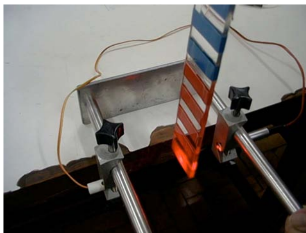
Figura 4 - Foto indicando a ponteira laser, o fotossensor e a placa bloqueadora.
