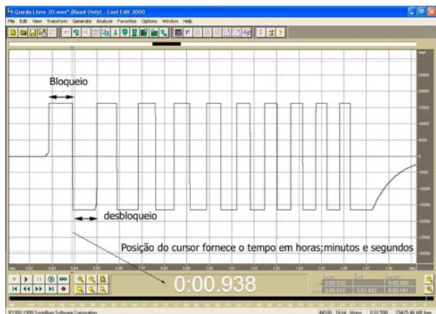
Figura 5 - Resultado obtido para o lançamento de uma placa entre o fotossensor e a ponteira laser, indicando os bloqueios e desbloqueios sucessivos produzidos. Cada instante de tempo pode ser obtido a partir da localização do cursor na tela.
