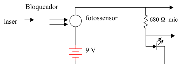
Figura 2 - Circuito utilizado para melhorar a relação sinal/ruído.
