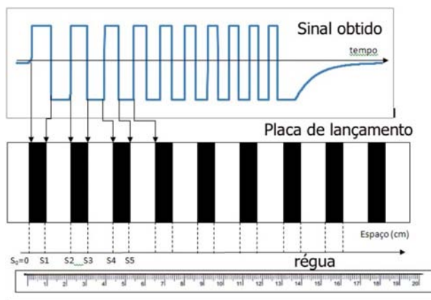
Figura 6 - Relação entre o sinal obtido através do programa de análise sonora e os intervalos de bloqueio de desbloqueio da placa de lançamento.
