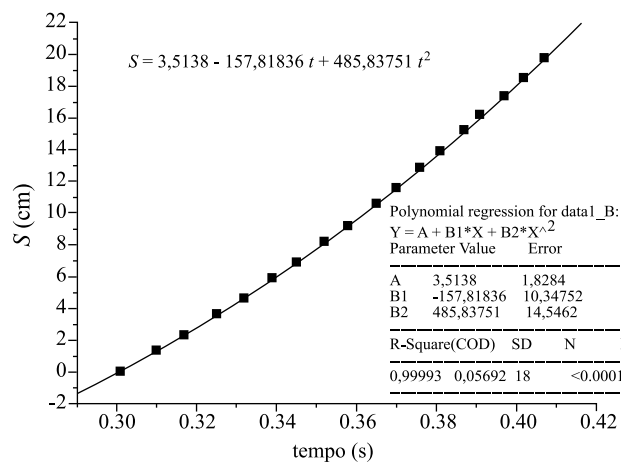
Figura 7 - Gráfico obtido para o lançamento de uma placa com fitas opacas previamente fixadas que permite bloqueios e desbloqueios de um fototransistor diretamente conectado à entrada de microfone de um PC. Uma tabela de posição vs. tempo é obtida a partir dos dados coletados em um programa de análise sonora.
