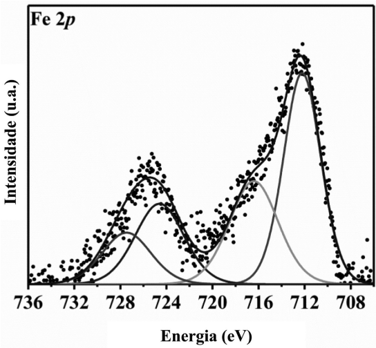
Figura 6: Espectro de Ferro de XPS com sobreposição de picos do meteorito Zagami.
