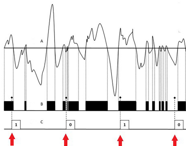
Figura 7: Esquema do processo de geração de números aleatórios utilizando o ruído de um diodo Zener. (A) A linha contínua representa o valor médio da tensão em uma janela de tempo definida. (B) O sinal amplificado é enviado a um circuito comparador que verifica se a tensão está acima ou abaixo do valor médio. (C) Em intervalos regulares, o circuito codifica o resultado em bits: 0 para tensões abaixo do valor médio e 1 para tensões acima.
