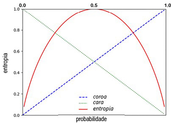
Figura 4: Entropia e probabilidade para a moeda.
