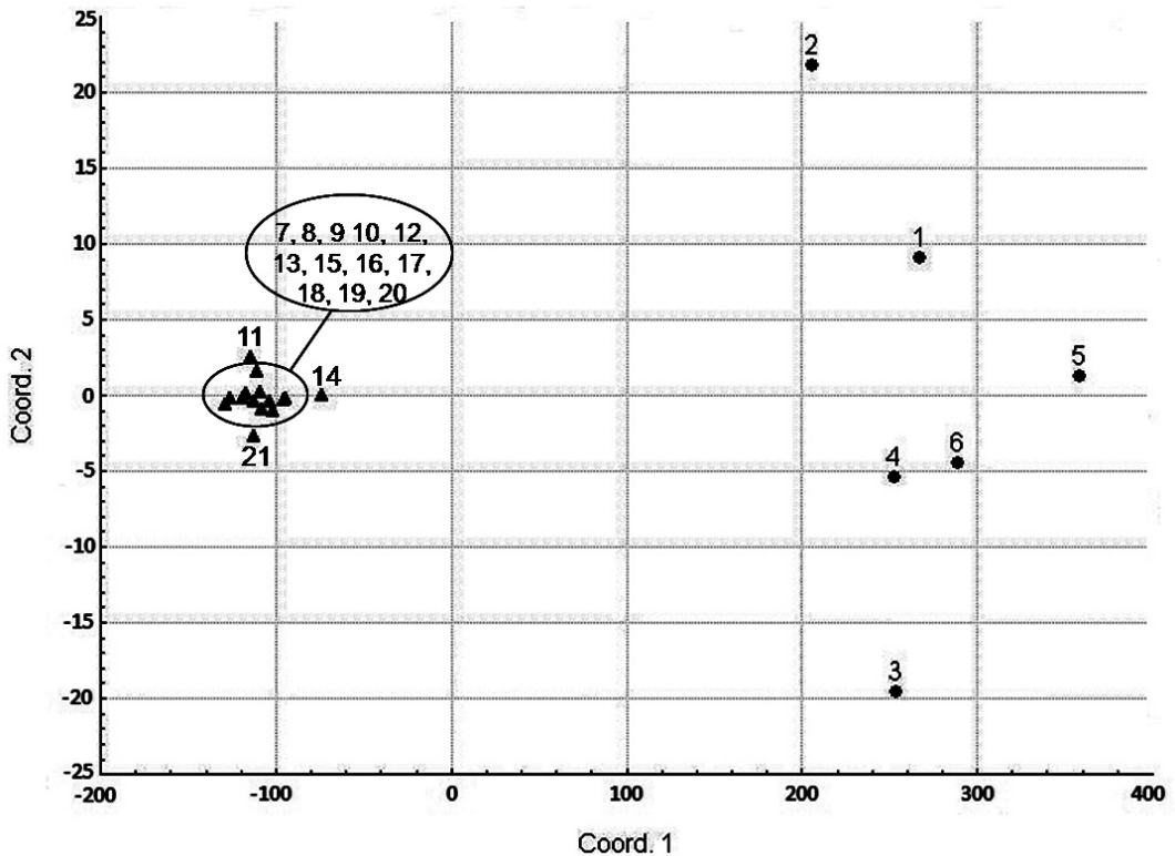
FIGURA 2 - Dispersão gráfica de 21 acessos de pitaya com base na matriz de Distâncias Euclidianas Médias Padronizadas calculadas, utilizando-se de onze características físico-químicas de frutos. ● = acessos de Hylocereus undatus (1 a 6), ▲ = acessos de S. setaceus (7 a 21). Os números 1 a 21 correspondem aos acessos descritos na Tabela 1.
