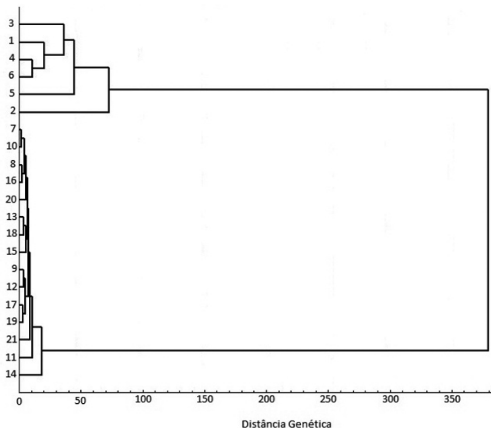
FIGURA 1- Análise de agrupamento de 21 acessos de pitaya com base na matriz de distâncias euclidianas médias padronizadas calculadas, utilizando-se de onze características físico-químicas de frutos. O método do UPGMA foi utilizado como critério de agrupamento. O valor do coeficiente de correlação cofenética ( r ) foi de 0,92. Os números 1 a 21 correspondem aos acessos descritos na Tabela 1.
