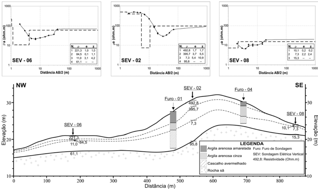
Figura 5 – Seção geoeletrica ao longo do perfil PG-06 (Fig. 4), baseado na interpretação das SEV's 02, 06 e 08 e informações geológicas dos furos 01 e 04.
