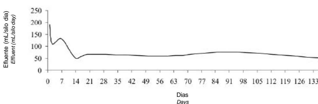
Figura 1 - Quantidade diária de efluente observada (mL) em um período de 136 dias de armazenamento, em silagens de capim-tanzânia não-emurchecido.
