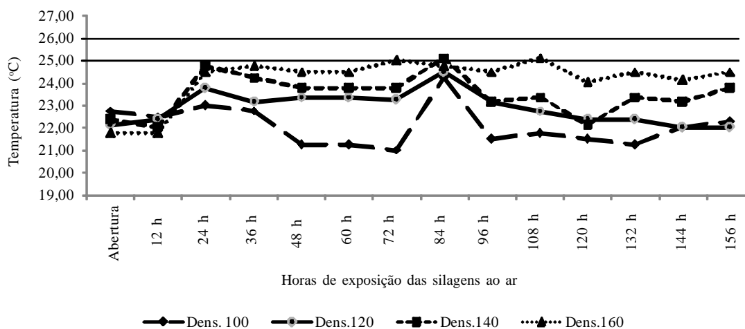
Figura 1 - Temperatura das silagens de capim-marandu submetidas a diferentes densidades na ensilagem ao longo do período de exposição aeróbia.
