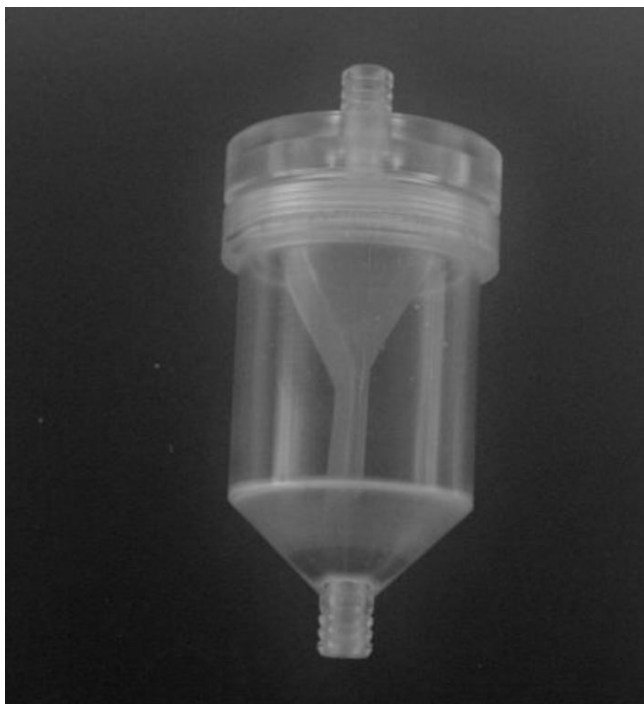
Figura 1 - Válvula unidirecional para drenagem pleural tubular fechada.
