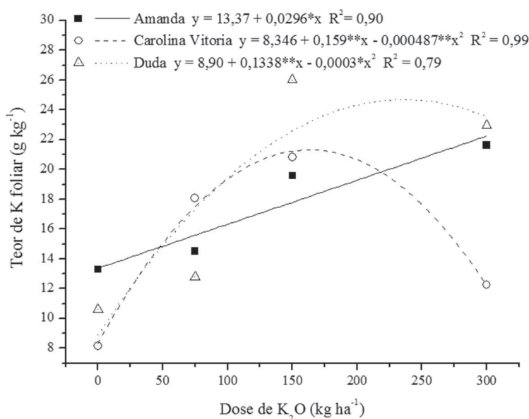
Figura 3. Curvas de resposta para teores foliares de K de três cultivares de batata-doce, aos 90 dias de cultivo, em função de doses de N, P 2 O 5 e K 2 O aplicadas ao solo. *, ** Coeficientes significativos a 5 e 1% de probabilidade pelo teste F, respectivamente.
