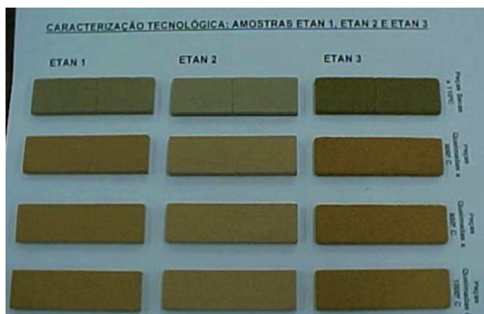
Figura 6 Caracterização tecnológica: peças secas a 110°C (A), peças queimadas a 900°C (B), 950°C (C) e 1.000°C (D).
