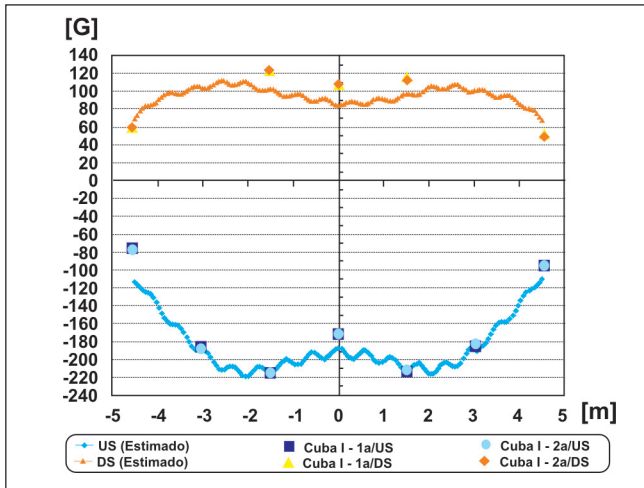
Figura 5 - Comparação entre B_x medido e calculado para a Cuba I.
