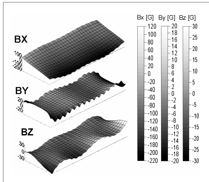
Figura 4 - Distribuições das 3 componentes de \vec{B} para a tecnologia ensaiada.
