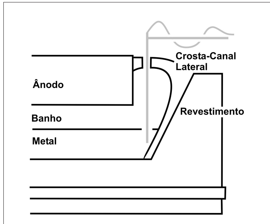
Figura 3 - Vista lateral do sensor em relação ao metal, ânodo e revestimento.
