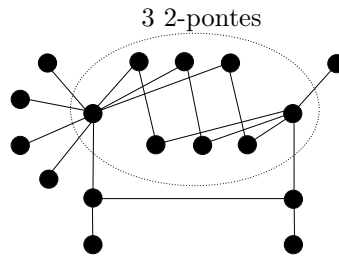
Figura 1: Grafo Z_3 -bem-coberto de cintura 6
