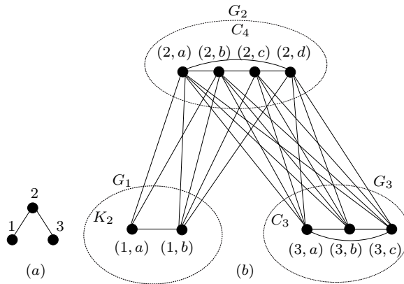
Figura 2: (a) Grafo P_3 e (b) Produto lexicográfico P_3 \circ \{K_2, C_4, C_3\}
