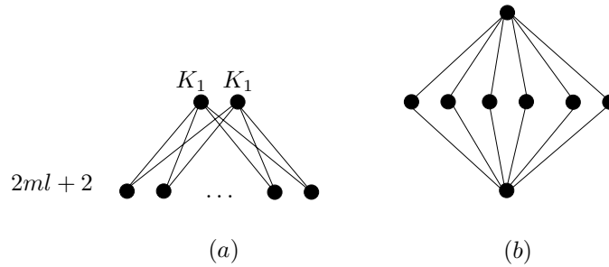
Figura 3: (a) Grafo K_{1,ml+1} \circ 2K_1 (b) Grafo K_{1,3} \circ 2K_1
