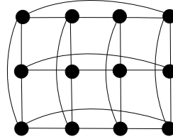
Figura 4: Grafo C_3 \times C_4
