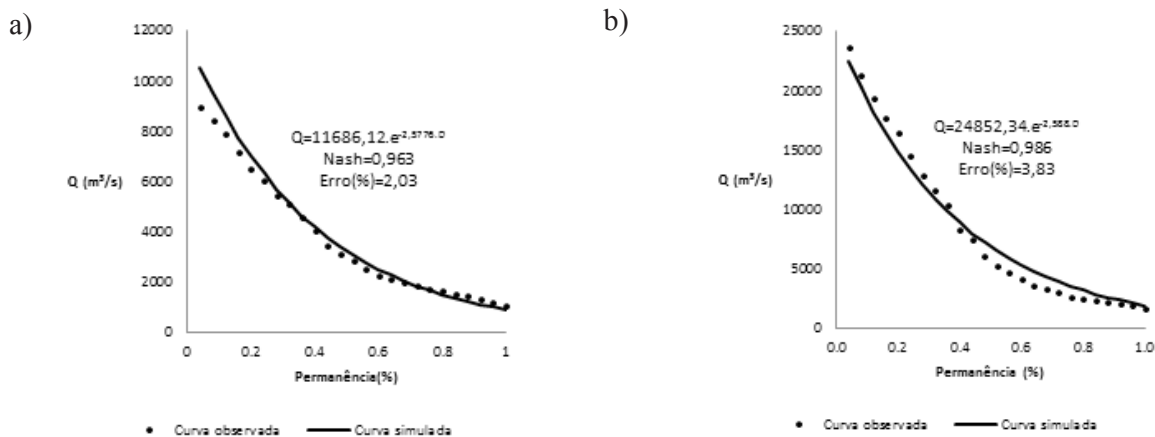
Figura 4 - Curvas de permanência observadas e simuladas para as bacias alvos da RHX.
